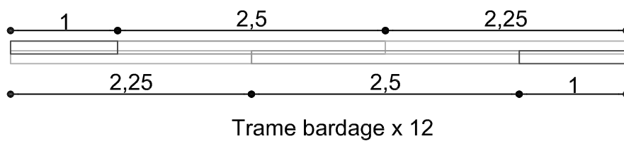
Façade Nord (façade bardée)
