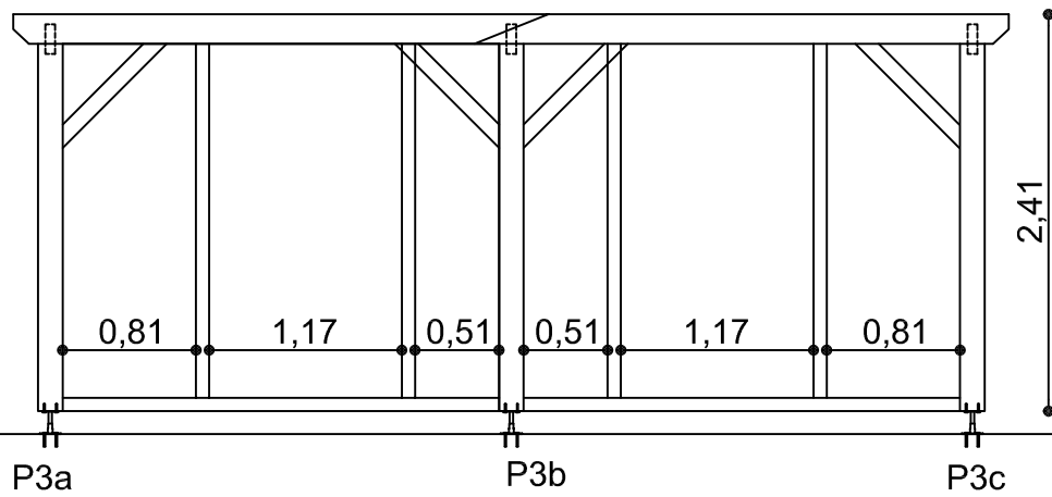
Façade Nord (façade bardée)
