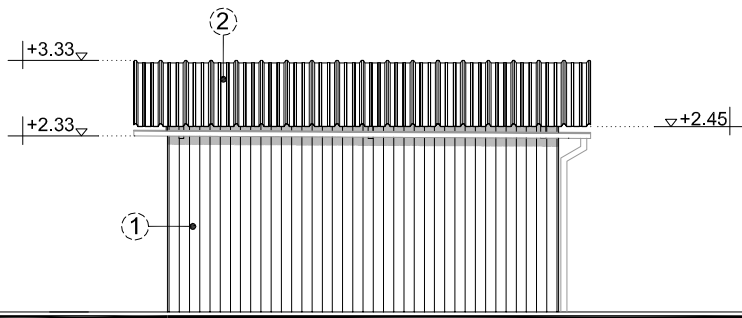
Façade Nord-Ouest
