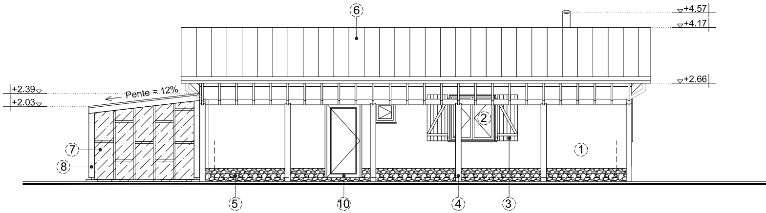
Façade Nord
